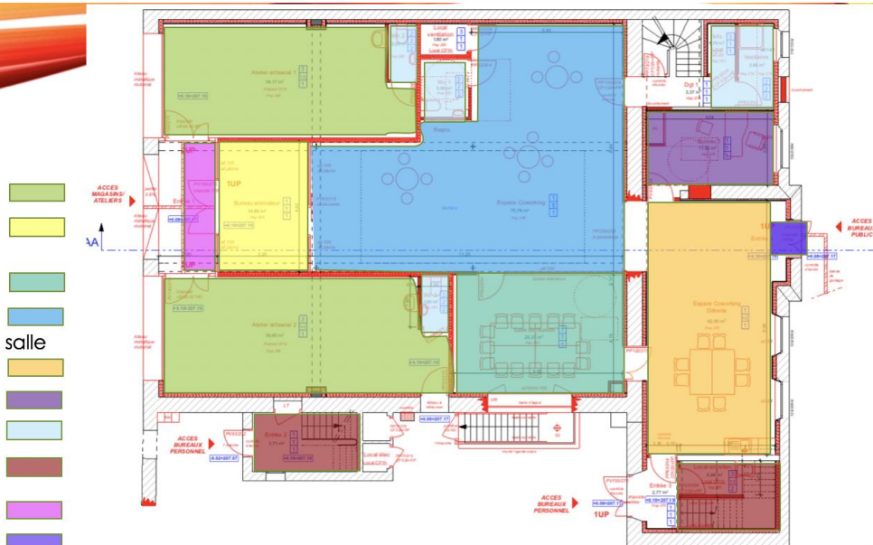
Existant
